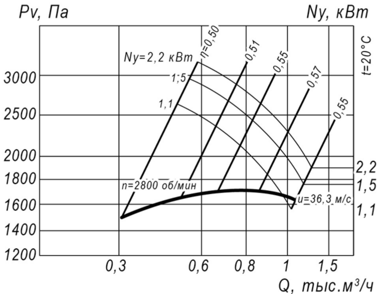
Аэродинамическая характеристика вентилятора ВР 12-26-2,5
